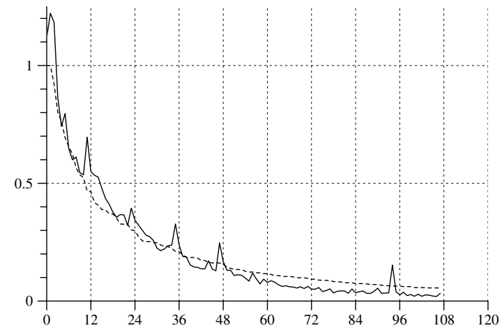
Abb. 13.1-7 Verteilung der bisherigen Bezugsdauern \alpha_{n97}(t) (durchgezogene Linie) und der Survivorfunktion G_{97}^* (gestrichelte Linie).
