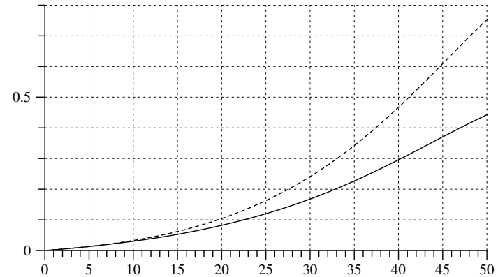
Abb. 14-6 Anteilsfunktion H^b (durchgezogene Linie) und Pseudo-Survivorfunktion 1 - \tilde{G}^b (gestrichelte Linie) für die Daten in Tabelle 14-4.
